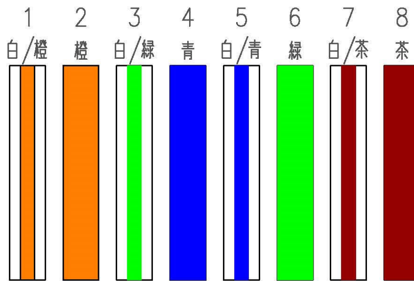
T568B 結線
