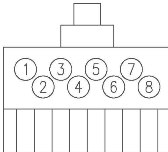
ピン配置 (差込側から見て)
